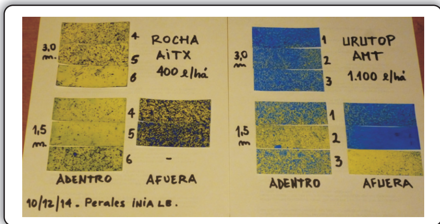
Figura 16: comparación de tarjetas hidrosensibles ubicadas sobre 3 plantas en 3 diferentes ubicaciones, luego de la aplicación con pulverizador de torre (izquierda) y axial común (derecha) (Zeballos y col, 2015).
