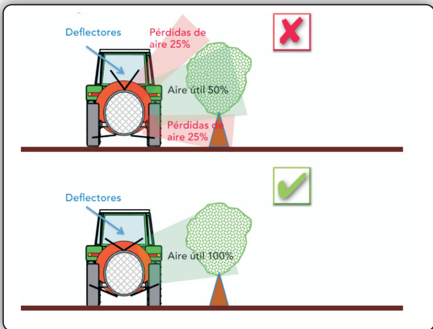
Figura 8: ajuste de la dirección del flujo de aire a la forma del cultivo (TOPPS Prowadis, 2014)
